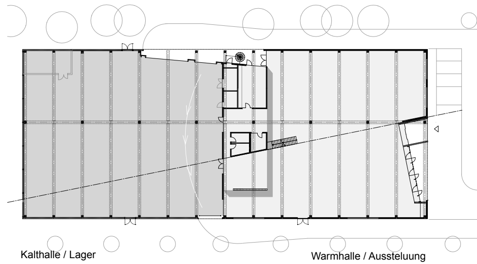
Grundriss o.M.
